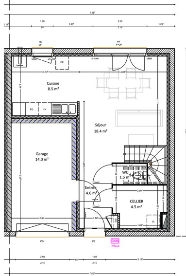
PLAN RDC
